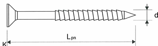
Rysunek A4. Tworzywowo-metalowe łączniki rozporowe EX \varnothing 8 S i CEX \varnothing 8 S
