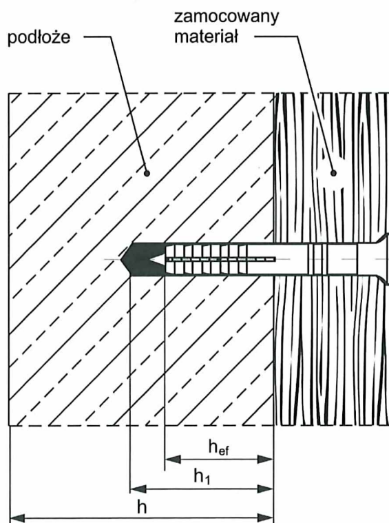
Rysunek B2. Parametry montażu łączników rozporowych EX \varnothing 6 S, EX \varnothing 8 S, CEX \varnothing 6 S i CEX \varnothing 8 S
