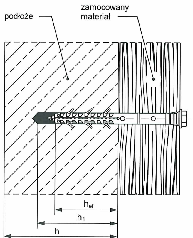
Rysunek B4. Parametry montażu łączników rozporowych PS ø10 i PS ø10 TP
