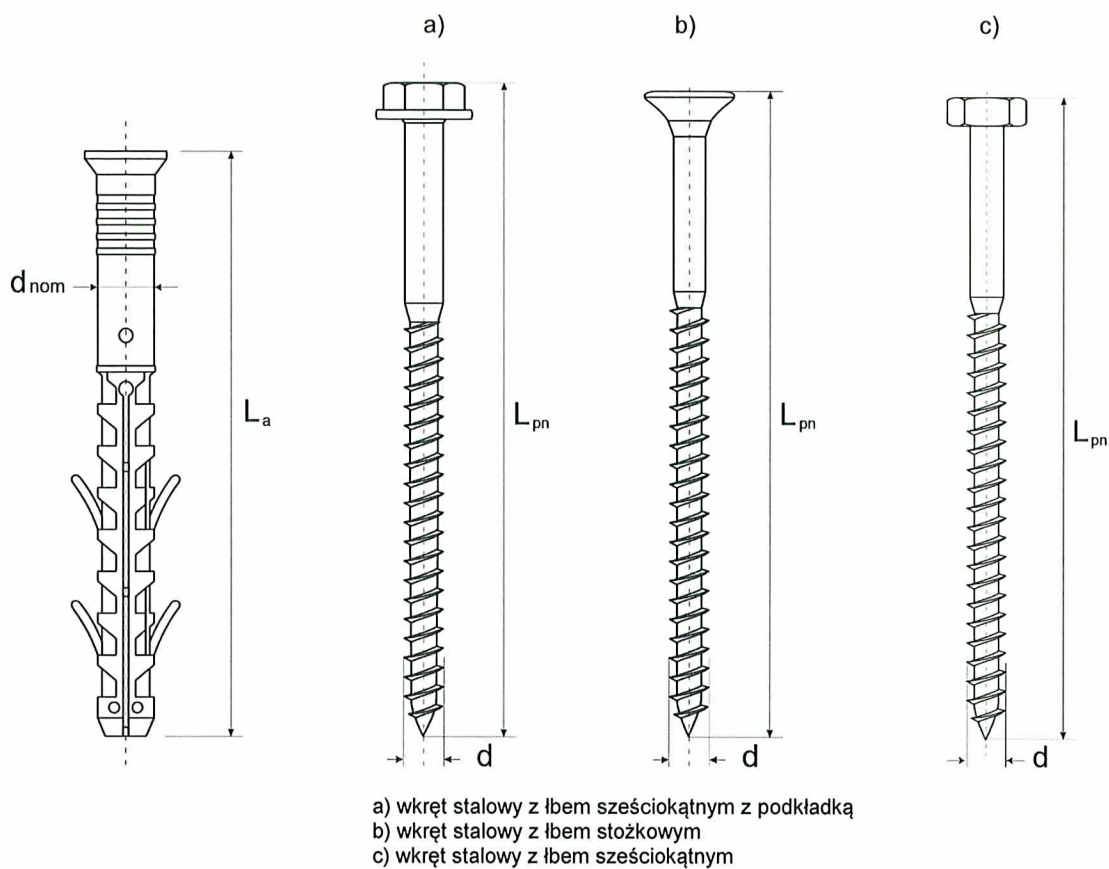
Rysunek A5. Tworzywowo-metalowe łączniki rozporowe PS ø8 TP, LS ø8 i PS ø8
