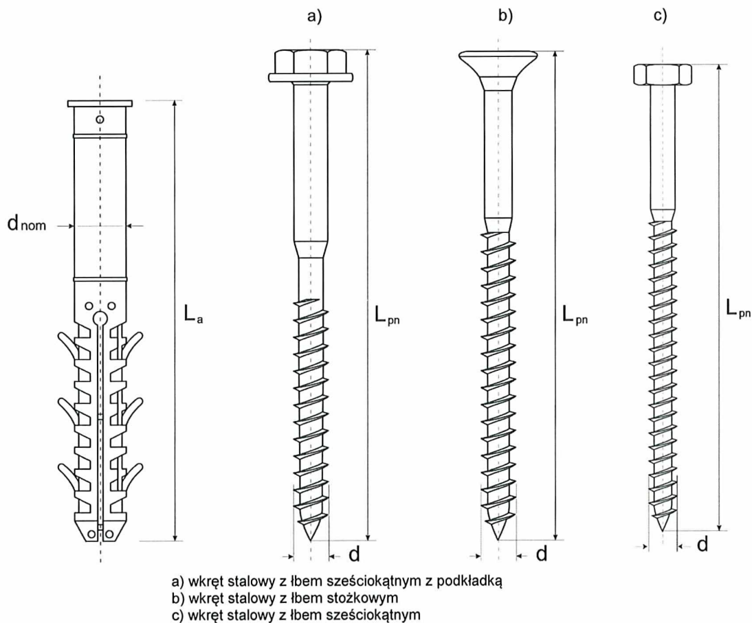
Rysunek A8. Tworzywowo-metalowe łączniki rozporowe PS \varnothing 14 TP, LS \varnothing 14 i PS \varnothing 14
