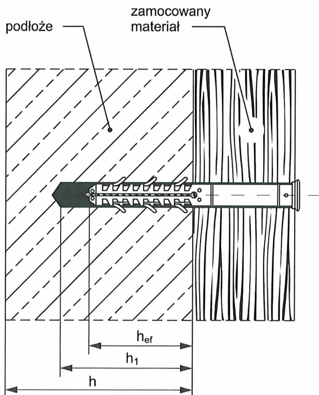
Rysunek B8. Parametry montażu łączników rozporowych LS ø12 i LS ø14
