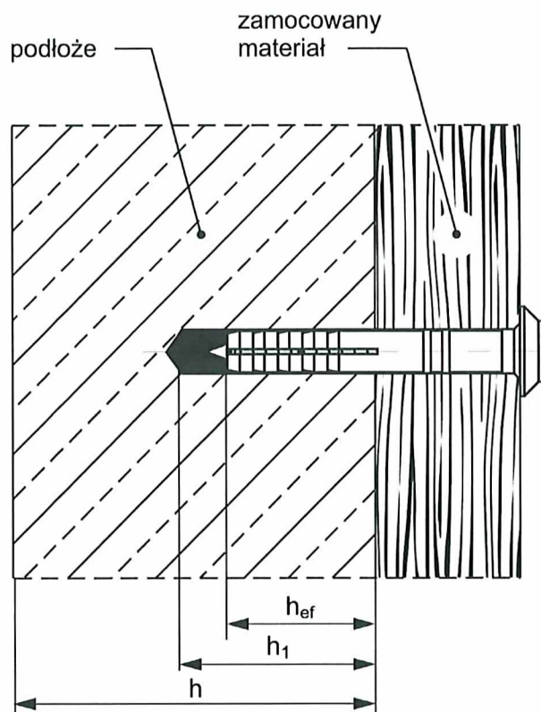
Rysunek B1. Parametry montażu łączników rozporowych EX \varnothing 6 K, EX \varnothing 8 K, CEX \varnothing 6 K i CEX \varnothing 8 K
