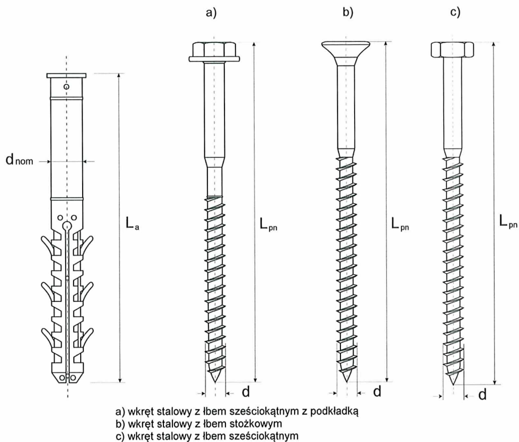
Rysunek A7. Tworzywowo-metalowe łączniki rozporowe PS \varnothing 12 TP i LS \varnothing 12 i PS \varnothing 12
