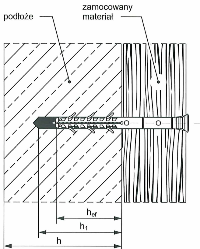
Rysunek B7. Parametry montażu łączników rozporowych LS ø10
