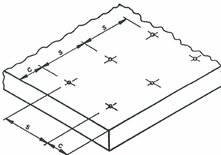
Rysunek B9. Parametry rozmieszczenia łączników rozporowych w podłożu
