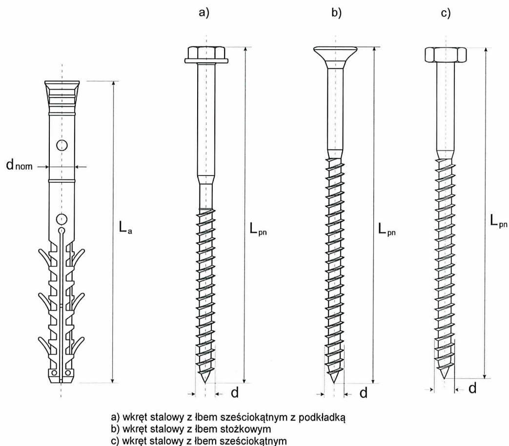
Rysunek A6. Tworzywowo-metalowe łączniki rozporowe PS ø10 TP, LS ø10 i PS ø10
