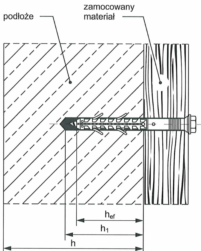
Rysunek B3. Parametry montażu łączników rozporowych PS ø8 oraz PS ø8 TP
