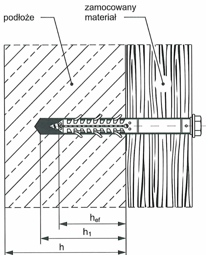
Rysunek B5. Parametry montażu łączników rozporowych PS \varnothing 12 , PS \varnothing 12 TP, PS \varnothing 14 i PS \varnothing 14 TP
